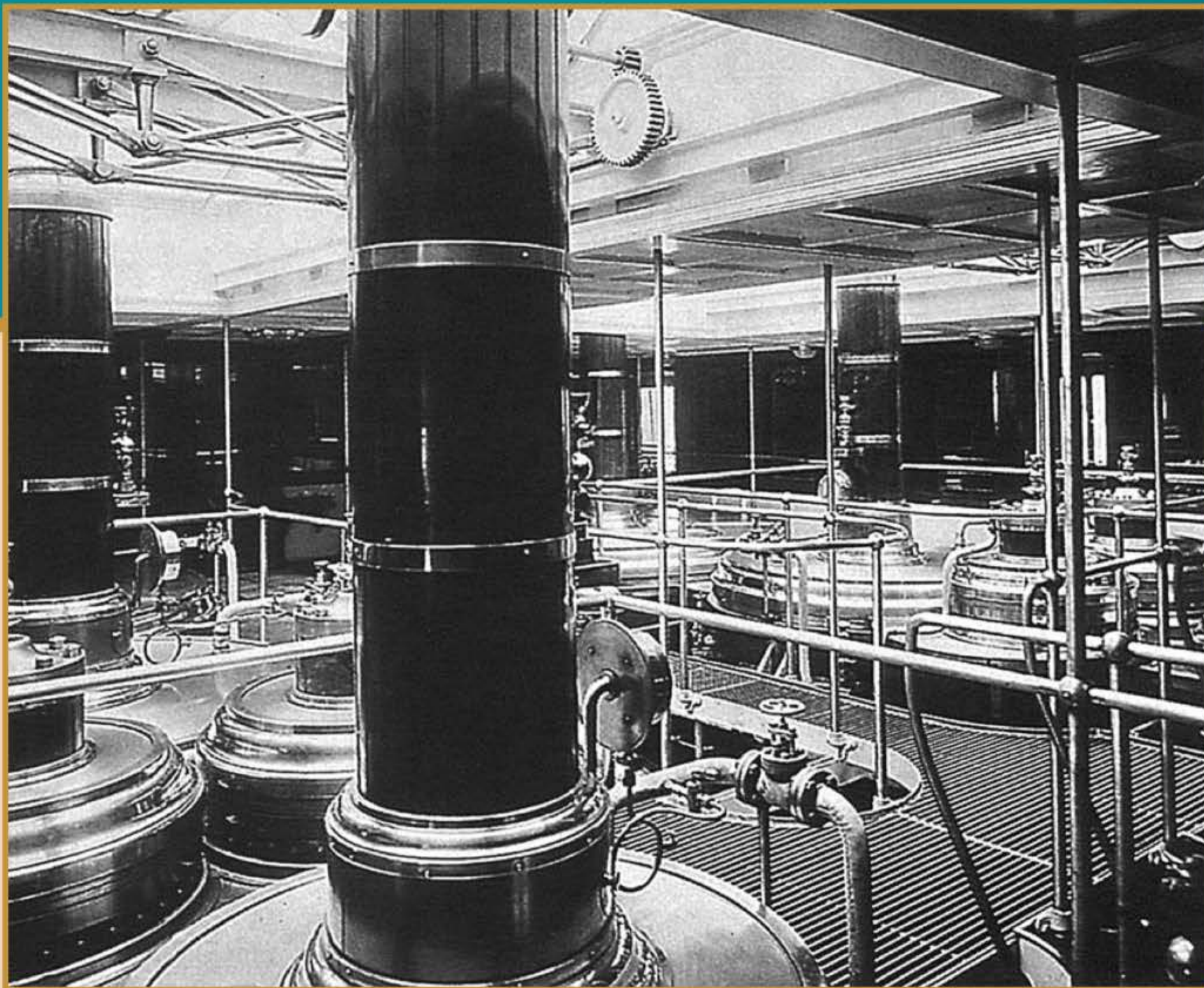
Паровая машина императорской яхты «Штандарт». Фотография 1890-х гг.
